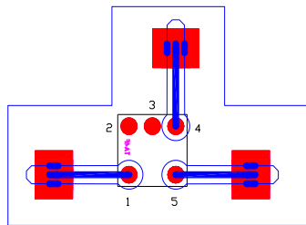
SCI-112F (Flip Chip)
