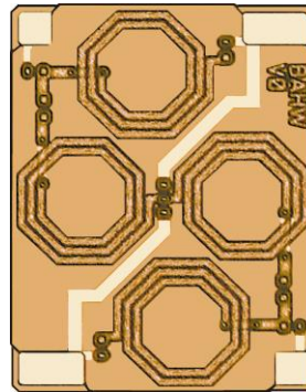
SCI-402W (Wirebond)
